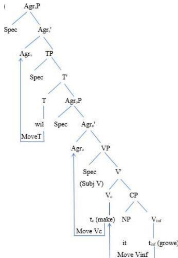
Рис. 1. Структура середньоанглійського речення з конструкцією AcI
