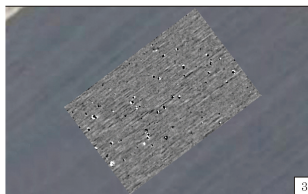
Рис. 6. Магнітні плани курганів, накладені на сателітну мапу Google: 1 — група Слобода Межирівська; 2 — група Токарівка, курган 4; 3 — група Токарівка, курган 6. Магнітний план підготував М. Пшибила, модифікував В. Рудь
