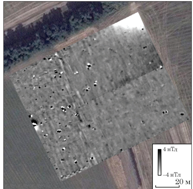
Рис. 3. Магнітний план кургану E групи Слобода Носковецька, накладена на сателітну мапу Google. Магнітний план підготував М. Пшибила, модифікував В. Рудь
