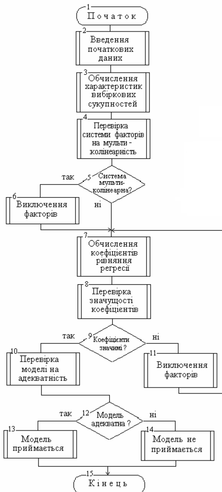
Рисунок 1 – Узагальнена блок-схема алгоритму побудови моделі
