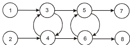
Рис. 1. Граф с контурами
