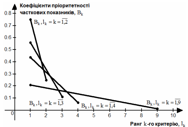
Рис. 2. Графік залежності коефіцієнтів пріоритетності часткових показників, розрахованих за методом Уея, від рангу k -го критерію
