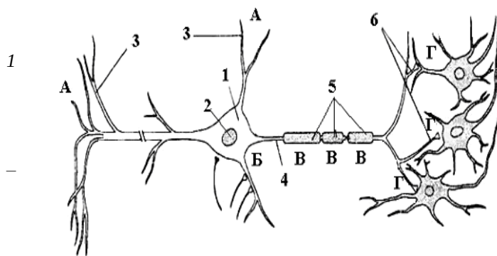
Мал.32. Схема будови нейрону та утворення контактів між ними:
