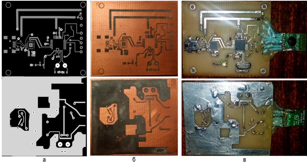
Рис. 7. Друкована плата аналізатора спектру на модулі CC2500: а — проект в графічному редакторі; б — витравлена; в — у готовому пристрою
