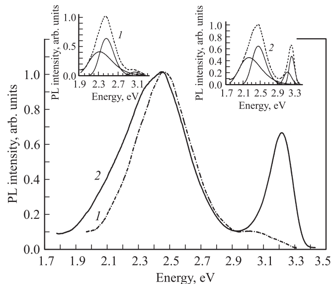
Рис. 2. Спектры фотолюминесценции (PL) пленки ZnO–Ag при 300 К в зависимости от условий приготовления: 1 — после легирования и окисления при температуре T_{\text{dop}} = 570^\circ\text{C} ; 2 — после отжига при температуре T_{\text{ann}} = 700^\circ\text{C} в течение 1 ч. Концентрация Ag > 3 ат%. На вставках показано разложение спектров 1 и 2 на гауссовы составляющие.
