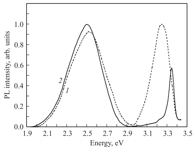
Рис. 3. Спектры фотолюминесценции (PL) пленки ZnO–Ag при 300 К (1) и 77 К (2). Легирование при T_{\text{dop}} = 570^\circ , отжиг при T_{\text{ann}} = 600^\circ\text{C} в течение 3 ч. Концентрация Ag > 3 ат%.
