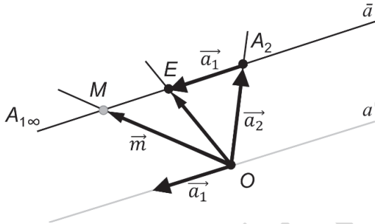
Рис. 2.2.9. Проективний репер на прямій із невласною фундаментальною точкою A_{1\infty} .
